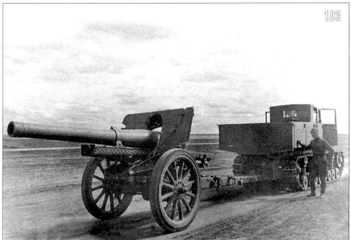
103. Тяжелый гусеничный советский тягач "Коминтерн" эвакуирует захваченное у японцев 150-мм орудие в тыл. Район реки Халхин-Гол, август 1939 года (АВЛ).
