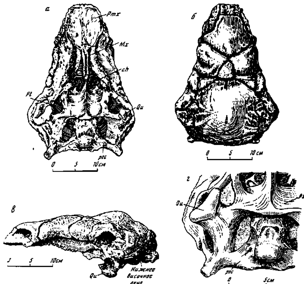
Рис. 1. Череп нодозавриды Panoplosaurus mirus Lambe. По У. Кумбеу (Coombes, 1978)
