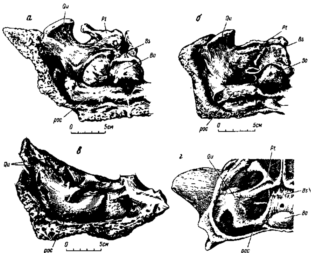
Рис. 6. Типы контакта квадратных костей с парокципитальными отростками у анкилозавридов а — тарбиян; б — шамозавр; в — шамозаврин, экз. ПИН, N 3779/1; г — сайханий (по: Maryanska, 1977) Обозначения см. на рис. 3
