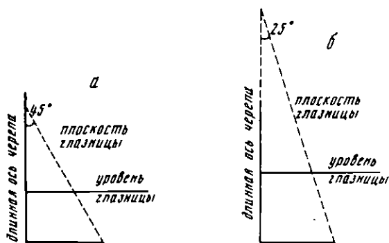
Рис. 15. Схема направленности плоскости орбит в черепе анкилозаврид а — шамозавр; б — тарих
