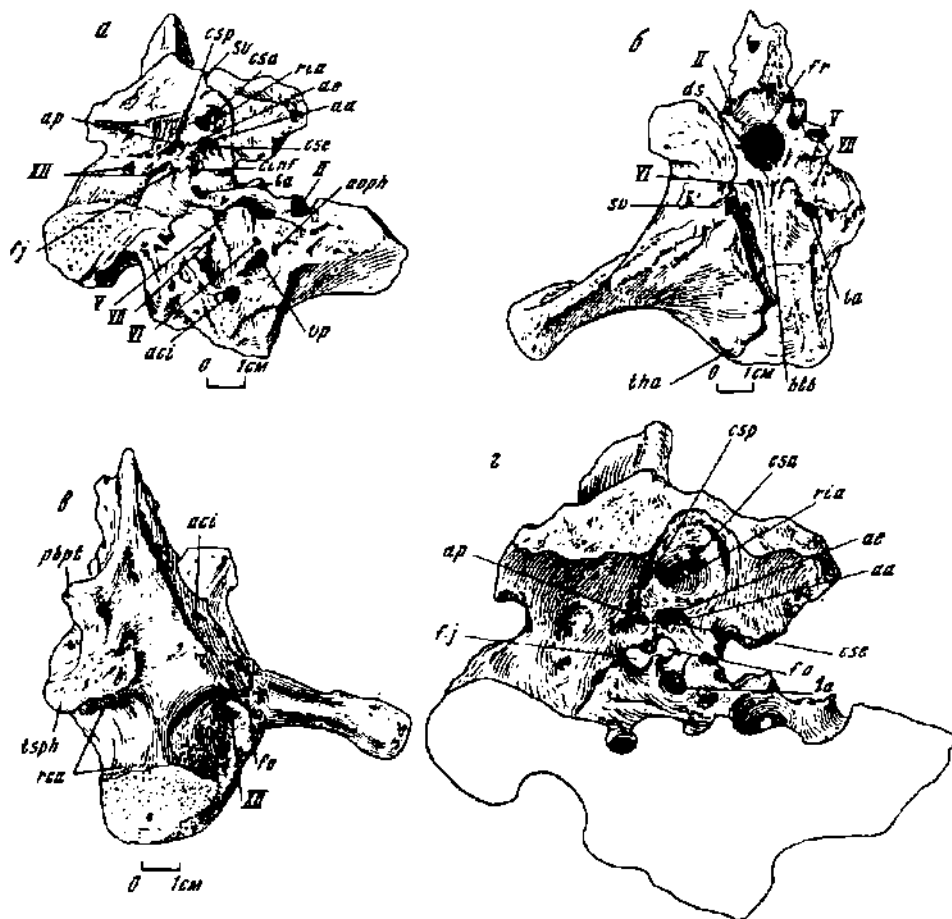
Рис. 7. Мозговая коробка анкилозауриды Talaururus plicatospineus Maleev. Экз. ПИН, N 3780/1; Байшин-Цав; верхний мел, байнширэнская свита
